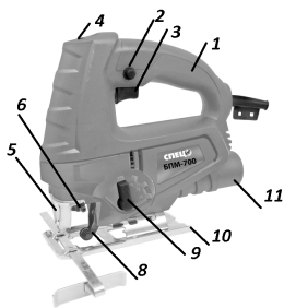
1. Корпус, 2. Фиксатор 3. Выключатель 4. Регулятор скоростных режимов 5. Защитный экран 6. Узел крепления пилки 8. Механизм качания пилки 9. Переключатель режимов маятникового хода 10. Опорная плита 11. Патрубок пылесоса
