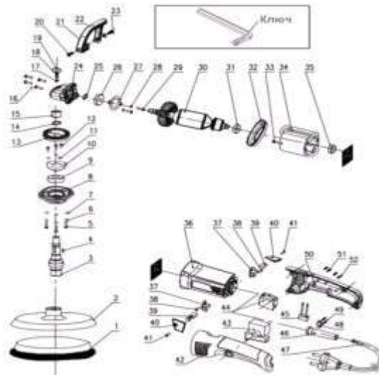
Рис.2 Схема разборки
