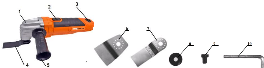
Рис.1. Общий вид
