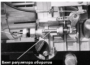
Рис. 7. Регулятор оборотов
